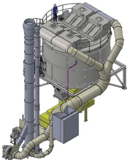
Projection 3D d'une partie du chantier
